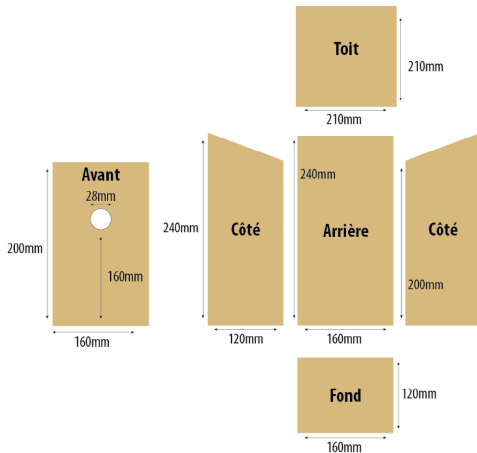
Plan d'un nidoir type boîte aux lettres pour les mésanges bleues
