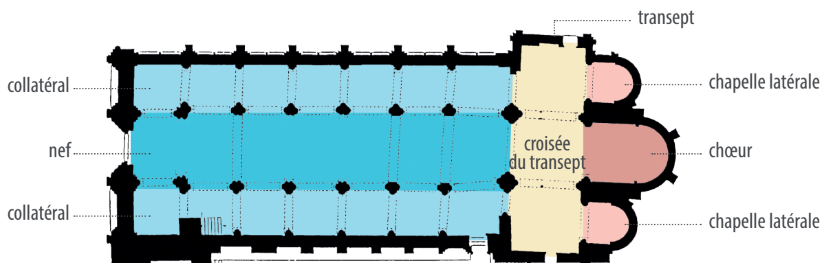
Plan de l'abbatiale Saint Vincent de Nieul-sur-l'Autise
