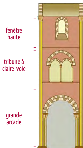
élévation d'une église romane
